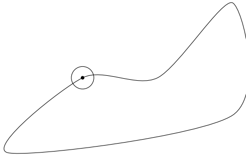
Abbildung 2.1: Randpunkt einer Menge M \subset \mathbb{K}^n
