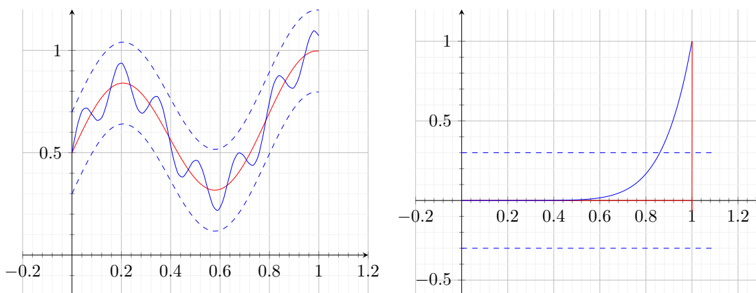
Abbildung 1.2: Links: „ \varepsilon -Schlauch“, Rechts: ?? (b) nicht gleichmäßig konvergent
