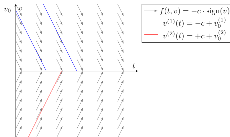
Abbildung 5.5: Mögliche Lösungen der DGL \dot{v} = -c \cdot \text{sign}(v) mit v_0^{(1)} > 0 und v_0^{(2)} < 0 . Ab t = \frac{v_0}{c} existiert keine Lösung.
