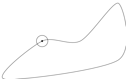
Abbildung 1: Randpunkt einer Menge M \subset \mathbb{K}^n
