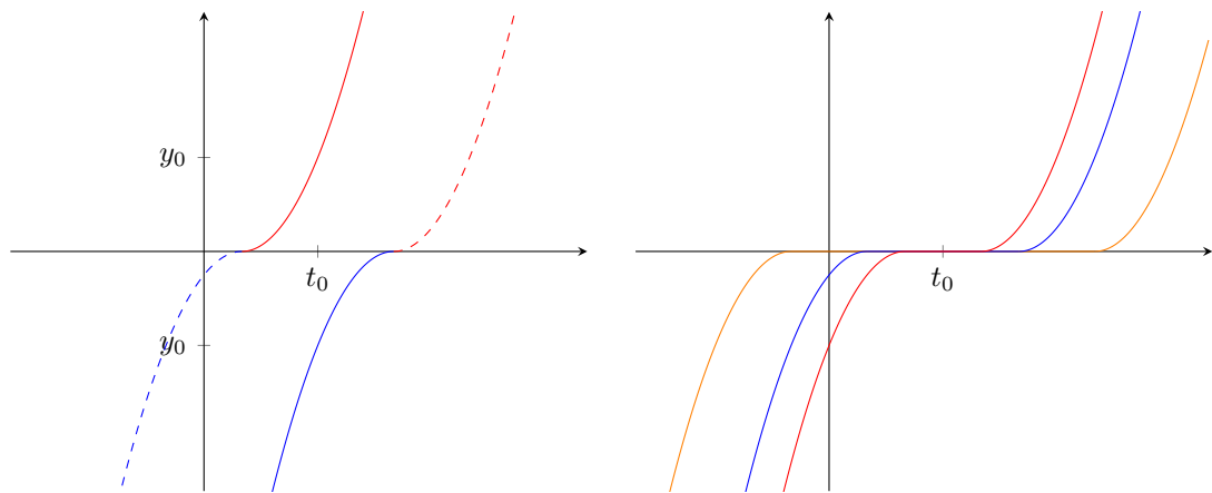
(a) Lösungen für y_0 > 0 (rot) bzw. y_0 < 0 (blau) und ihre Fortsetzungen. (b) Für y_0 = 0 existieren beliebig viele zusammengesetzte Lösungen.
