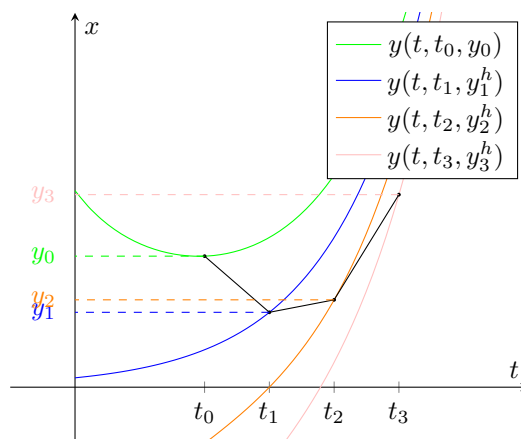
Abbildung 5.2: Eulersches Polygonzugverfahren
