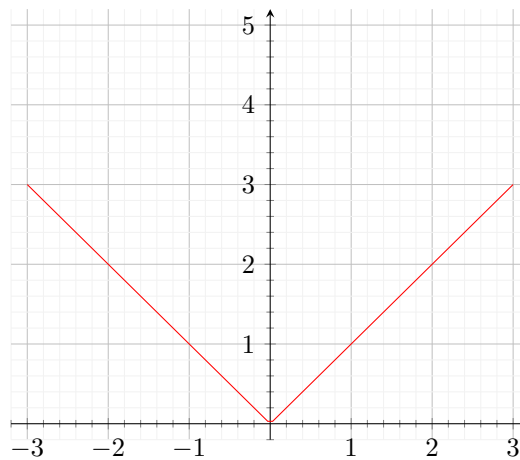
Abbildung 5.2: Betragsfunktion
