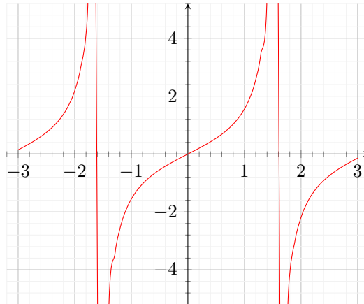
Abbildung 4.1: \tan(x)
