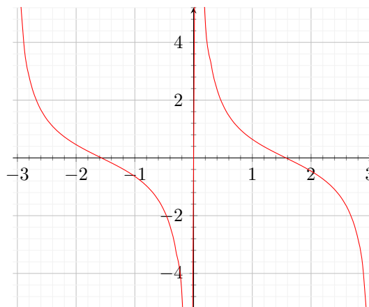
Abbildung 4.2: \cot(x)
