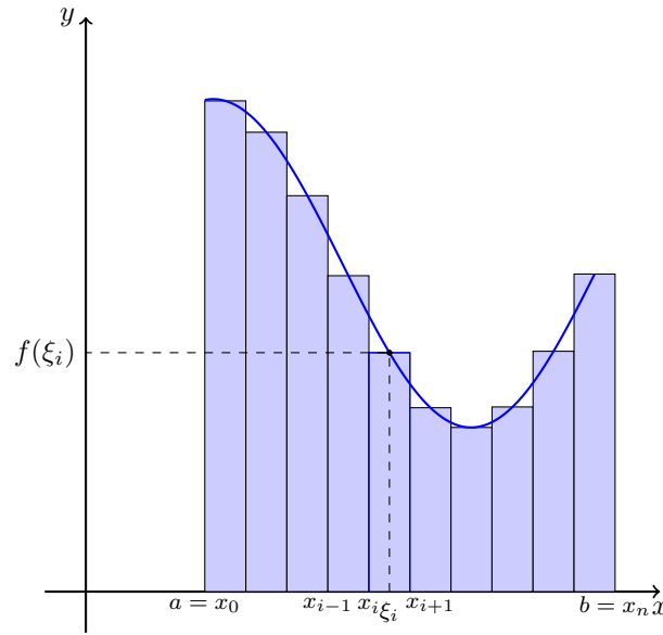
Abbildung 6.1: Riemannsche Summen
