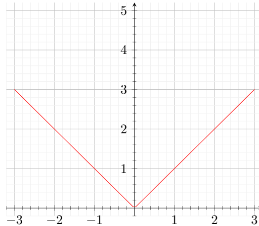
Abbildung 4: Betragsfunktion
